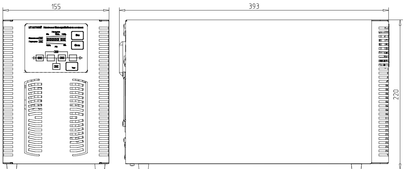
Рисунок 1.1 – Внешний вид ИБП Штиль ST1101L (AT1) Габаритные размеры и внешний вид
